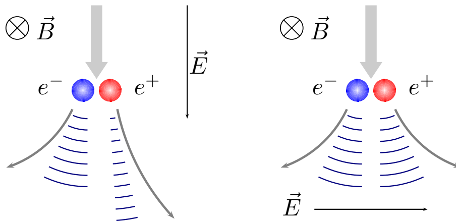
Abbildung 3.3: Veranschaulichung des Einflusses der unterschiedlichen Orientierungen des elektrischen Feldes auf die Radioemission eines Elektron-Positron-Paares.
