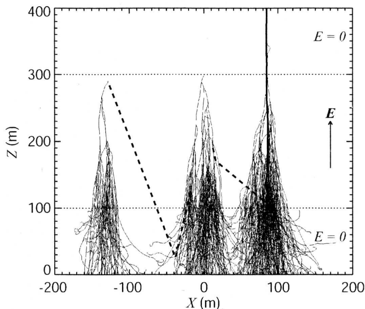
Abbildung 6.8: Simulation zum Auftreten einer relativistischen Rückkopplung während des Runaway Breakdowns durch Bremsstrahlungsphotonen oder rückwärtsgestreuter Positronen [Bet09]. Die Simulation wurde mit einem 1 MeV Elektron gestartet, das oben in der Mitte in einen Bereich mit einer Feldstärke von 1000 \text{ kVm}^{-1} eintrat. Links und rechts davon sind beispielhaft die zwei möglichen Arten der Rückkopplung dargestellt.
