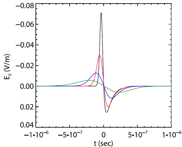
Abbildung 6.9: Simulierte Radiopulse eines Runaway Breakdowns, die durch einen Luftschauer mit einer Energie von 10^{17} eV und einer Einfallsrichtung von 45^\circ relativ zur Senkrechten hervorgerufen werden. Die Feldstärken für die berechneten Pulse sind 250 \text{ kVm}^{-1} , 375 \text{ kVm}^{-1} , 625 \text{ kVm}^{-1} und 1250 \text{ kVm}^{-1} . Die Antenne befindet sich nahe des Luftschauerzentrums am Boden, wobei die Region mit der hohen Feldstärke in einer Höhe von 5 Kilometern liegt [Dwy09].
