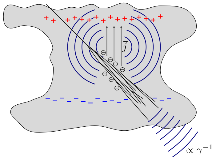
Abbildung 3.4: Veranschaulichung der Strahlungscharakteristik des Geosynchrotroneffekts mit dem zusätzlichen Strahlungsbeitrag durch die erzeugten Ionisationselektronen in einer Region hoher Feldstärke, wie zum Beispiel einer Gewitterwolke. Die Stromdichte \vec{j} führt in erster Näherung zu einer dipolartigen Abstrahlung.
